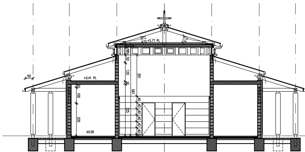
PREREZ 1
