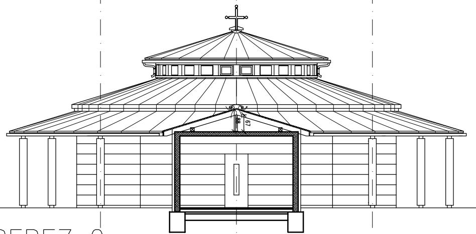
PREREZ 2
